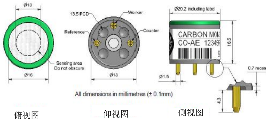
图1 CO-AE示意图
