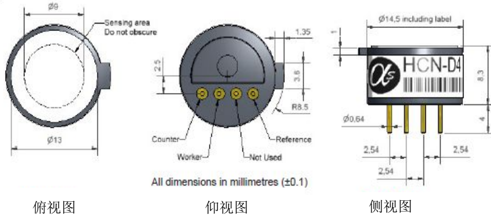
图1 HCN-D4 示意图
