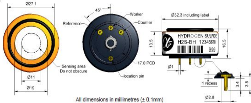
俯视图
