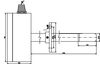
外形尺寸图
