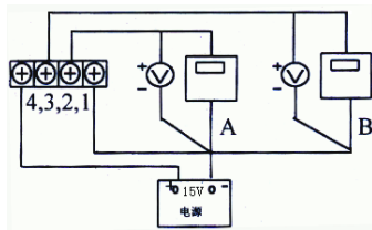
RH30B-V 接线图
